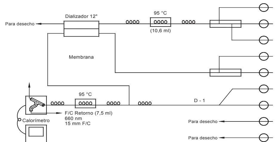
Figura 3. Autoanalizador usado en la determinación de fosfatos”
